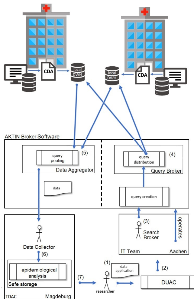
Abbildung 2: Architekturübersicht
